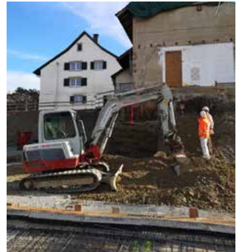
Unterfangung in Etappen von denkmalgeschütztem Objekt
